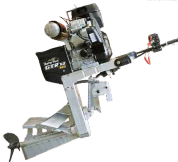
GATORTAIL GTR37XD EFI MOTOR
